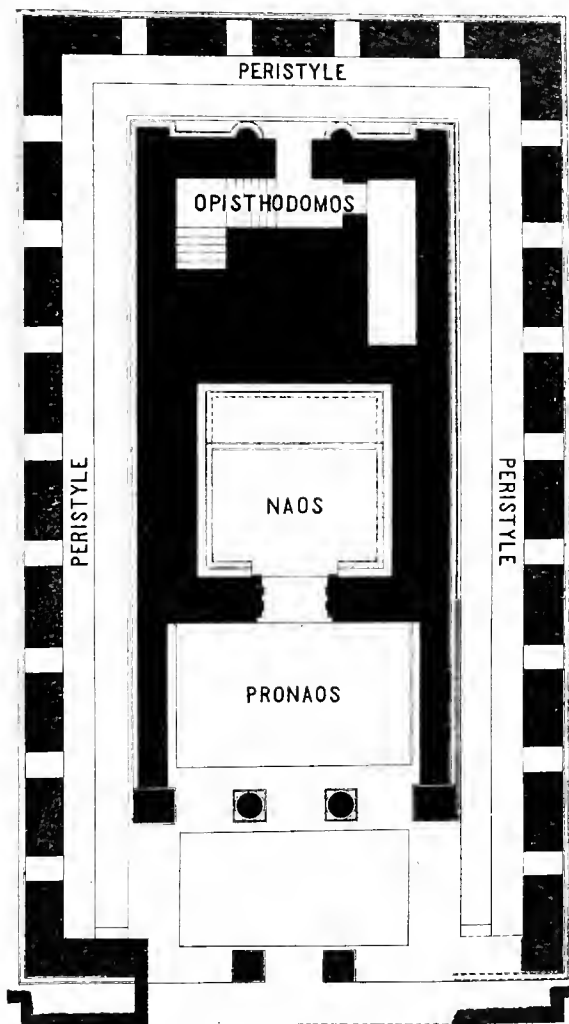
JANDIAL TEMPLE: PLAN.
